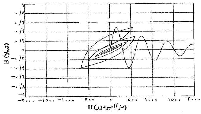
شکل ۱۸- منحنی پسماند هسته به ازای موج سینوسی میراشونده زمانی برای چگالی القایش مغناطیسی هسته
