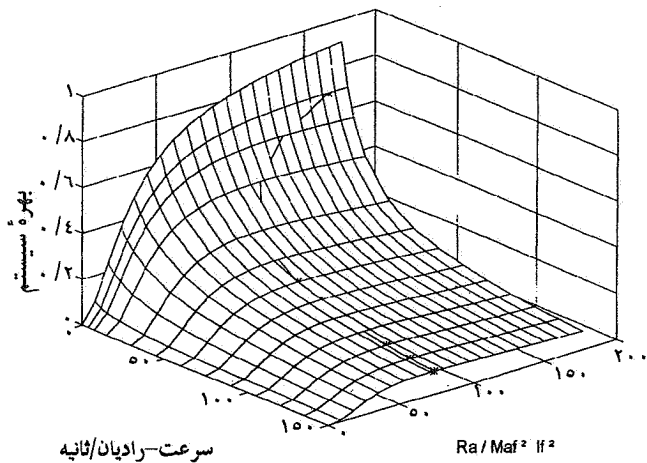
شکل ۲۲- بهره سیستم در موتور تحریک جداگانه حداکثر آندرسرعت ثابت: -۰-
