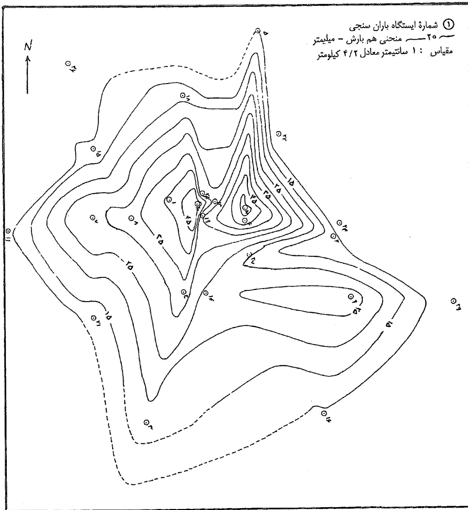
شکل ۲- خطوط هم باران باران ۷۱/۳/۱۶ مشهد
