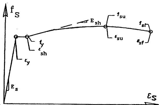
شکل ۳- منحنی تنش- کرنش و مقادیر مشخصه روی منحنی فولاد معمولی
