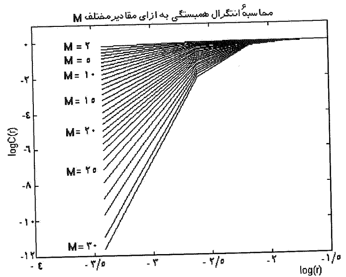
شکل (۲): منحنیهای \text{Log}(C_M(r)) بر حسب \text{Log}(r) به ازای مقادیر M از ۲ تا ۳۰
