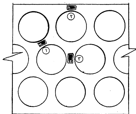
شکل ۸- محل نصب کرنش‌سنجها روی ورقهای در وسط تیر
