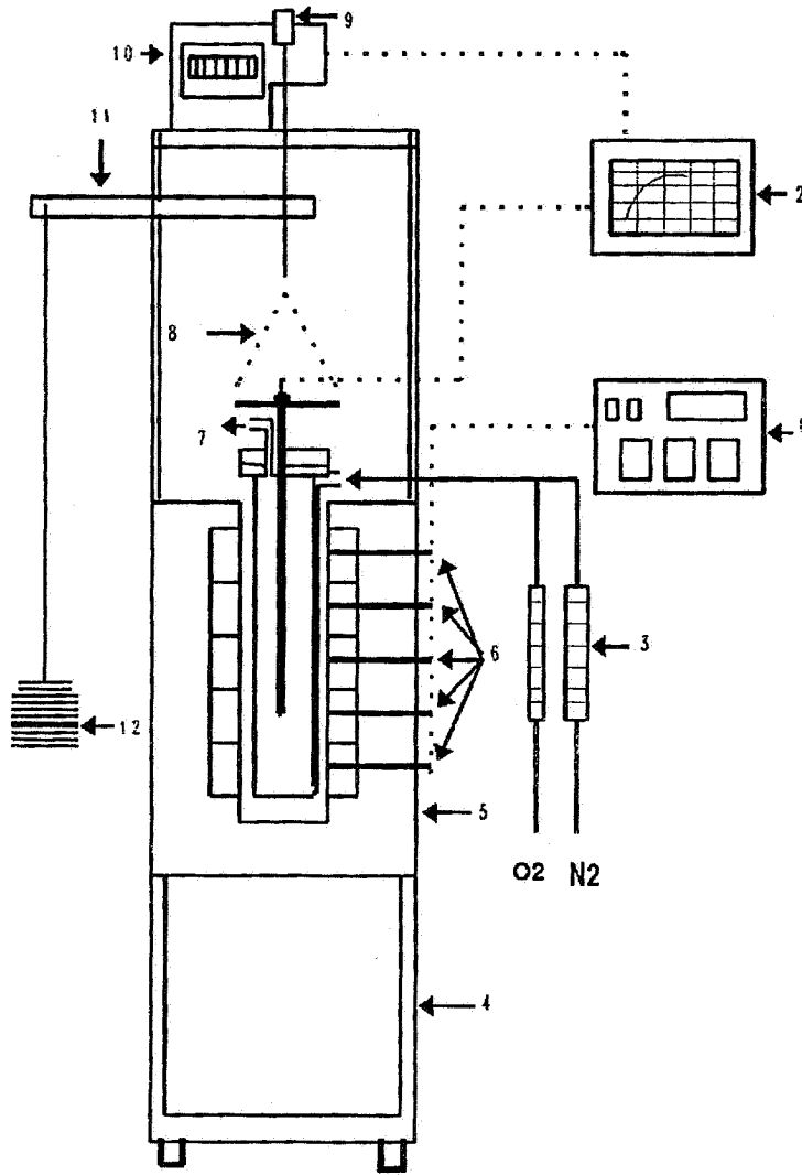
شکل ۱- شماتیک دستگاه ترموگراویمتری
