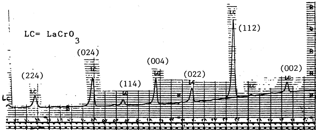
شکل ۳- الگوی پراش پرتو X ترکیب لانتانیوم کرومیت کلوغه شده در دمای 1100^\circ\text{C}
