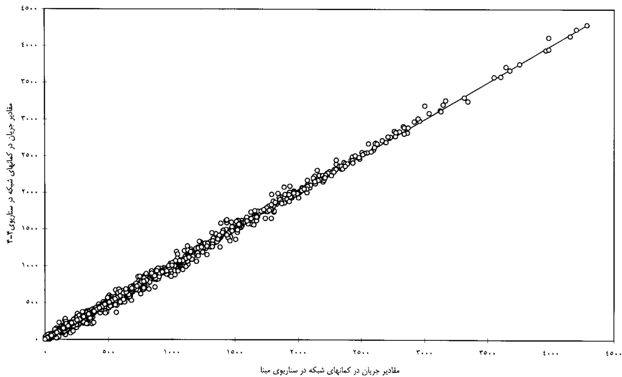
شکل ۷- نمودار پراکنده‌گی جریان در کمانهای شبکه در سناریوی ۴-۴ نسبت به سناریوی مبنا
