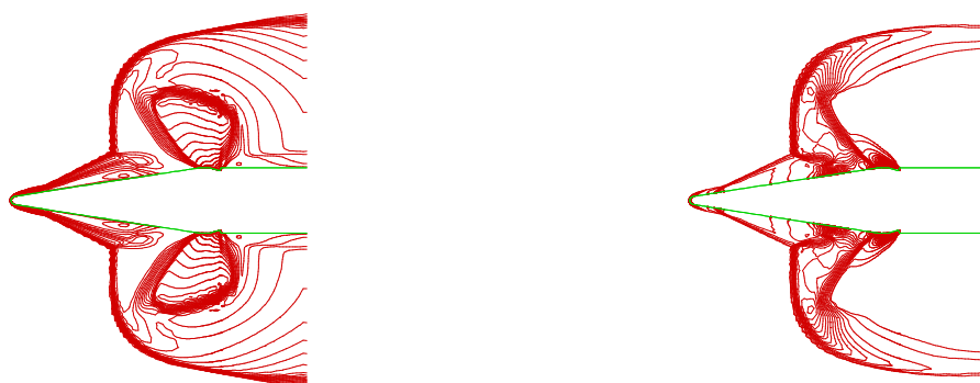
خطوط همتراز عدد ماخ
