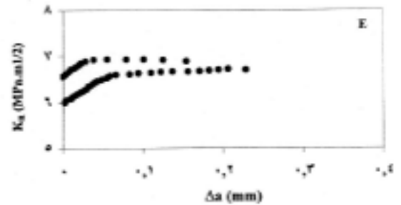
شکل ۶- منحنیهای R برای نمونه‌های D و E و منحنی نیرو - جابه‌جایی برای نمونه B
