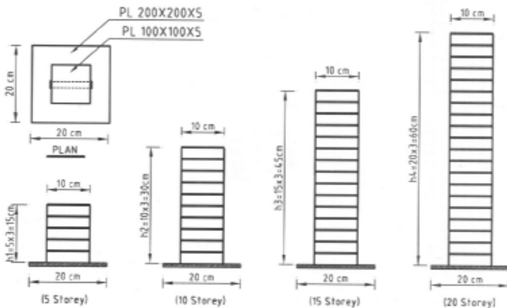
شکل ۸- مشخصات مدل‌های سازه ای ۵، ۱۰، ۱۵، ۲۰ و ۲۰ طبقه
