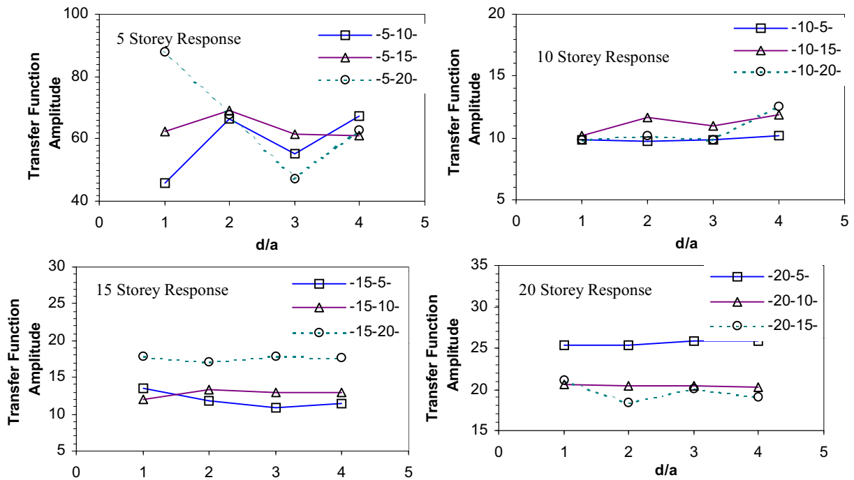
شکل ۲۲- تغییرات حداکثر دامنه پاسخ شتاب نوک مدل‌های سازه‌های مجاور هم در مد اول بر حسب نوع و فاصله سازه‌ها تحت زلزله الاسترو
