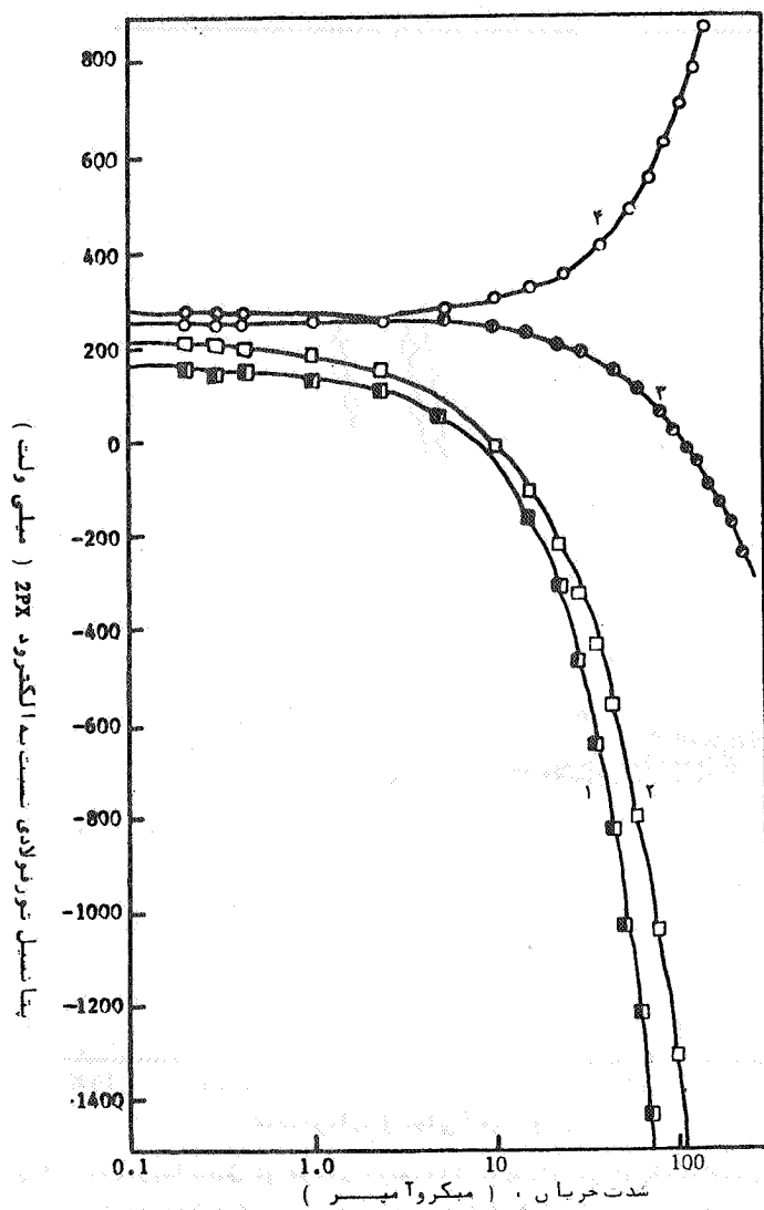
شکل ۴ تغییر پتانسیل تورنسیل به آهن تورنسیل در مقابل شدت جریان برای پلاریزاسیون کاتدی صفحه فولادی . منحنی‌های ۴۰۳،۲۰۱ بر ترتیب پتانسیل تورنسیل در موقعیت ۴۰۳،۲۰۱ نسبت به الکترود 2PX در موقعیت ۴ را نشان میدهد .
