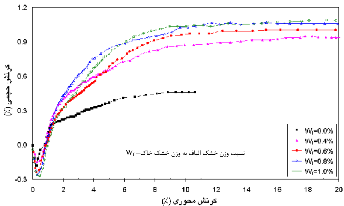
شکل ۵- تغییرات تنش انحرافی (شکل الف) و کرنش حجمی (شکل ب) در آزمایش سه محوری CD ( s'_c = 100 kPa ) برای درصدهای
