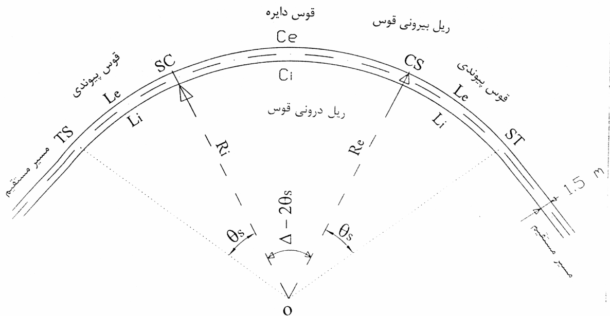
شکل ۵ - پارامترهای هندسی قوسهای ریل بیرونی و درونی
