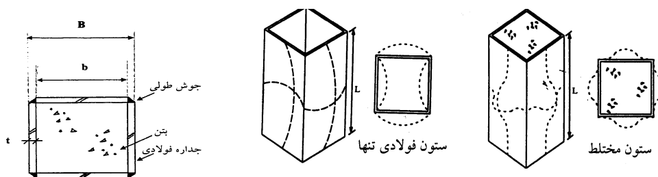
شکل ۲- مقطع عرضی سکون
