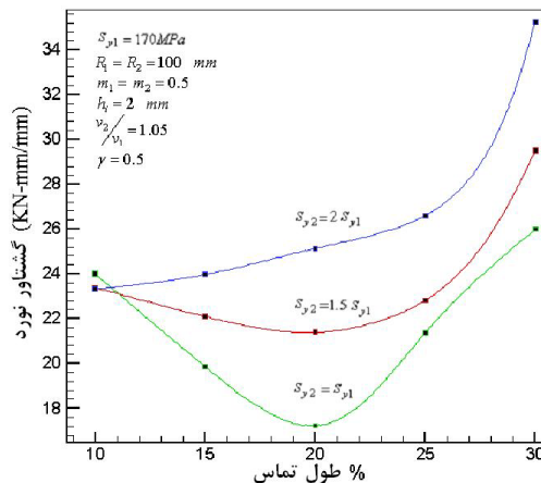
شکل ۱۴- تغییرات گشتاور مورد نیاز بر اساس کاهش در ضخامت‌های مختلف و نسبت‌های مختلفی از تنشهای مختلفی از تنشهای تسلیم دو لایه ورق
