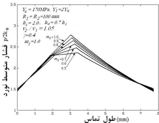
شکل ۱۷- چگونگی توزیع فشار متوسط بر اساس تغییرات
