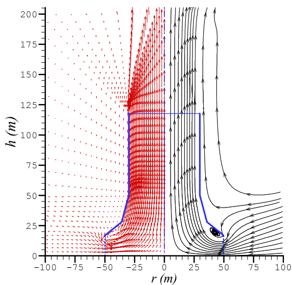
شکل ۸- میدان سرعت و خطوط جریان داخل و خارج برج خنک کننده خشک طبیعی
