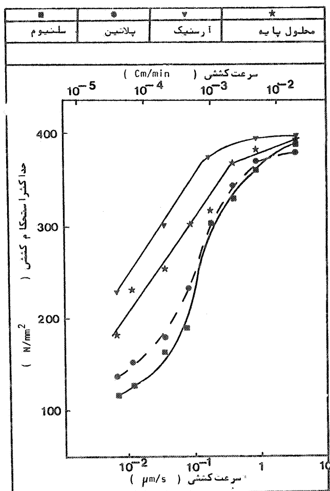
شکل ۶: تا شير سرعت کشش و نوع سموم کاتدی ( غلظت 25ppm ) اضافه شده به محلول پایه بر استحکام کشش
