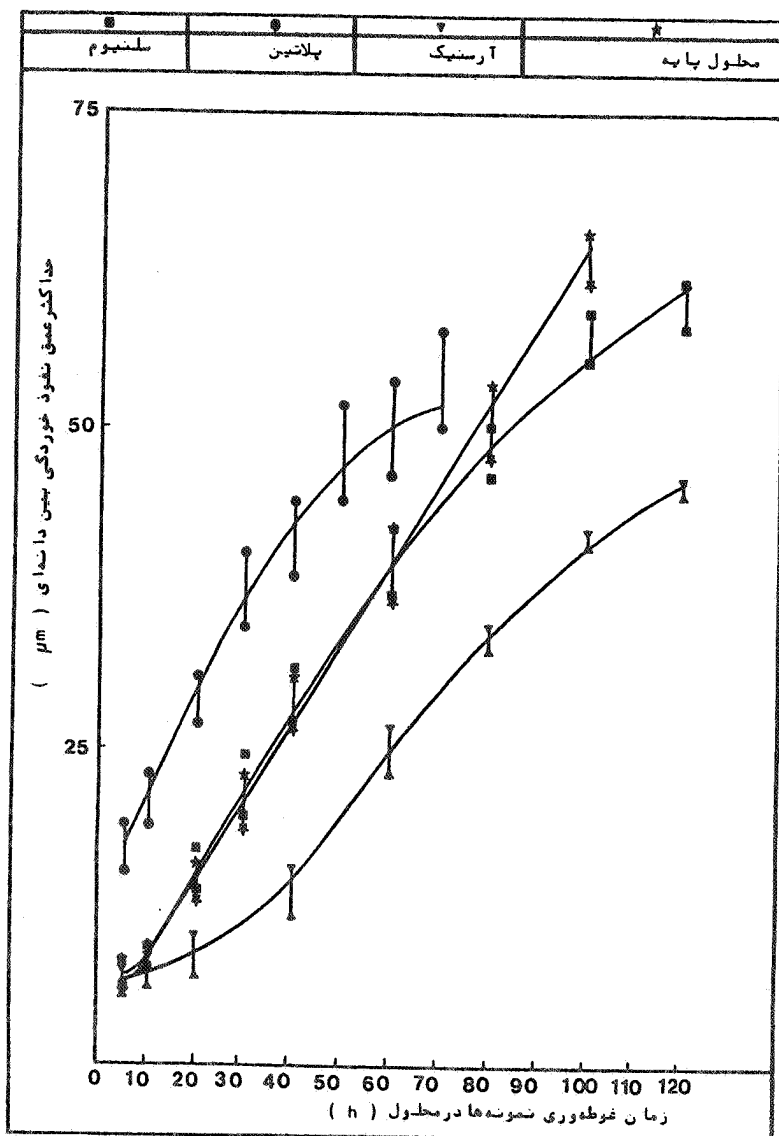
شکل ۱۱ : تأثیر زمان غوطه‌وری بر حداکثر عمق نفوذ خوردگی بین دانه‌ای در محلول پایه و محلول پایه حاوی 25ppm آرسنیک از نمونه‌ها در محلول مختلف.
