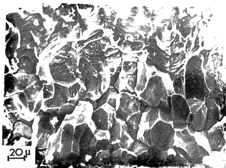
شکل ۱۰ : تصویر میکروسکوپی الکترونی از سطح مقطع شکست نمونه‌های غوطه‌ور شده در محلول، شامل خوردگی بین دانه‌های درکناره‌ها و شکست مکانیکی نسردر بقیه نمونه .
