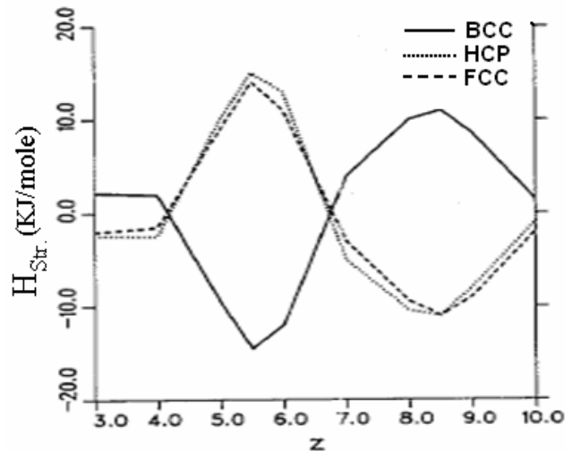
شکل ۹- انتالپی فلزات واسطه بر حسب الکترونهاي ظرفیتی z در ساختارهای کریستالی متفاوت [۳۰]
