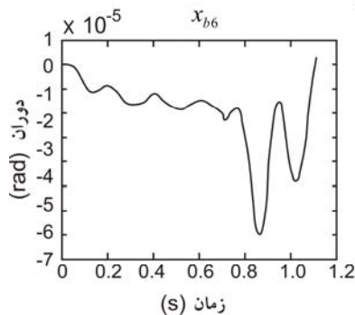
شکل ۱۲- انتقال قائم (پرش) و دوران قاب بوژی برای یک مدل بوژی کامل عبوری از تکه مرکزی
