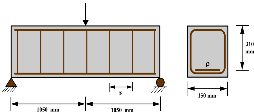
شکل ۱۷- مشخصات هندسی و مکانیکی تیر B 7
