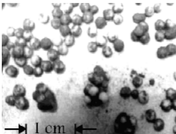
شکل ۹- نمایی از توزیع نایکنواخت ذرات SiC روی دانه‌های فومی، پیش از قالبگیری
