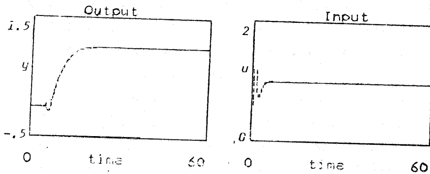
شکل ۱۹- پاسخ نسبت به تغییر پله‌ای واحد در y_r با کنترل کننده \bar{IMC} با وجود محدودیت در ورودی (مثال ۲)
