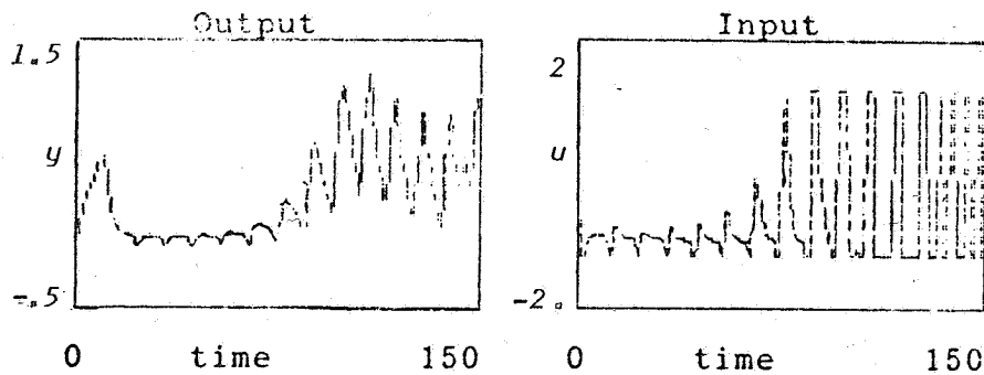
شکل ۱۳- پاسخ نسبت به تغییر d برای کنترل کننده پس‌خور معادل IMC با وجود محدودیت در ورودی بدون آنتی‌وا ایندآپ (مثال ۱)
