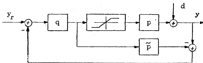
شکل ۵- دیاگرام IMC با اعمال محدودیت به فرآیند تنها
