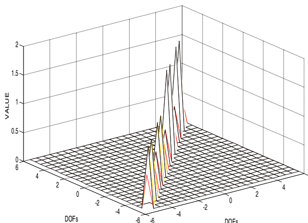
شکل ۱۰- ماتریس جرم مدل المان محدود اولیه سازه جکتی
