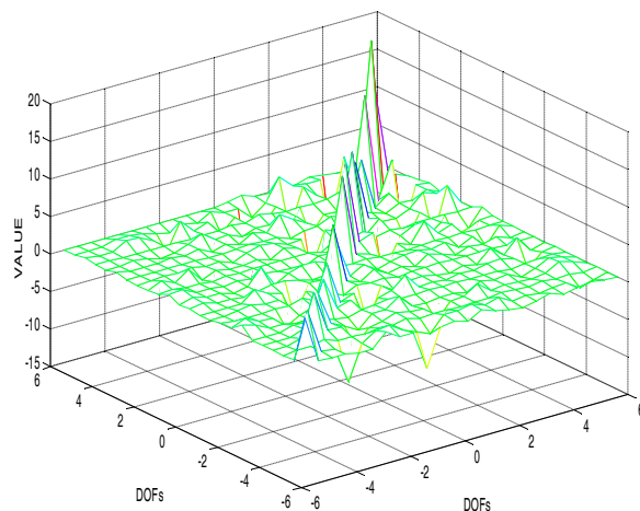
شکل ۱۳- خصوصیات ماتریس جرم به روزرسانی شده بر اساس ماتریس بردار ویژه اندازه گیری شده در روش مستقیم لاگرانژی
