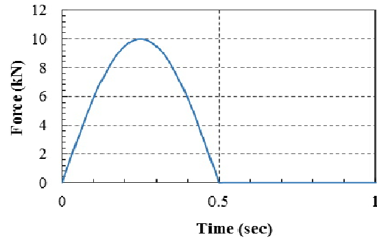
شکل ۶- تغییرات بار P_1 در حوزه زمانی
