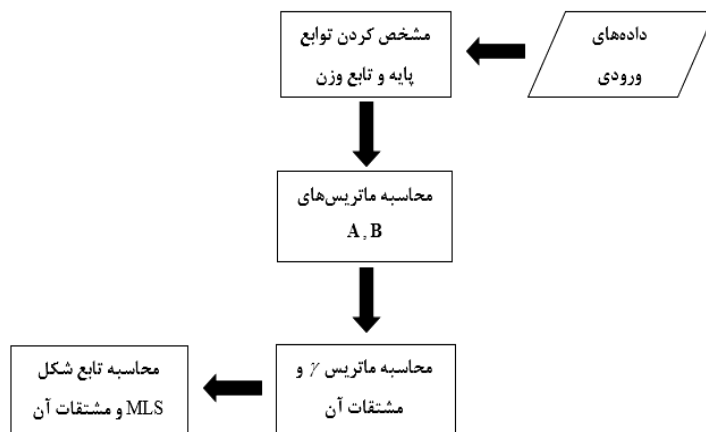
شکل پ ۱. فلوچارت روش محاسبه تابع شکل MLS
