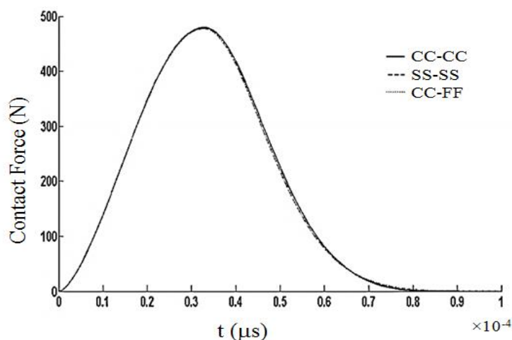
شکل ۸- تغییرات نیروی تماس در مرکز صفحه 50 \times 50 mm
