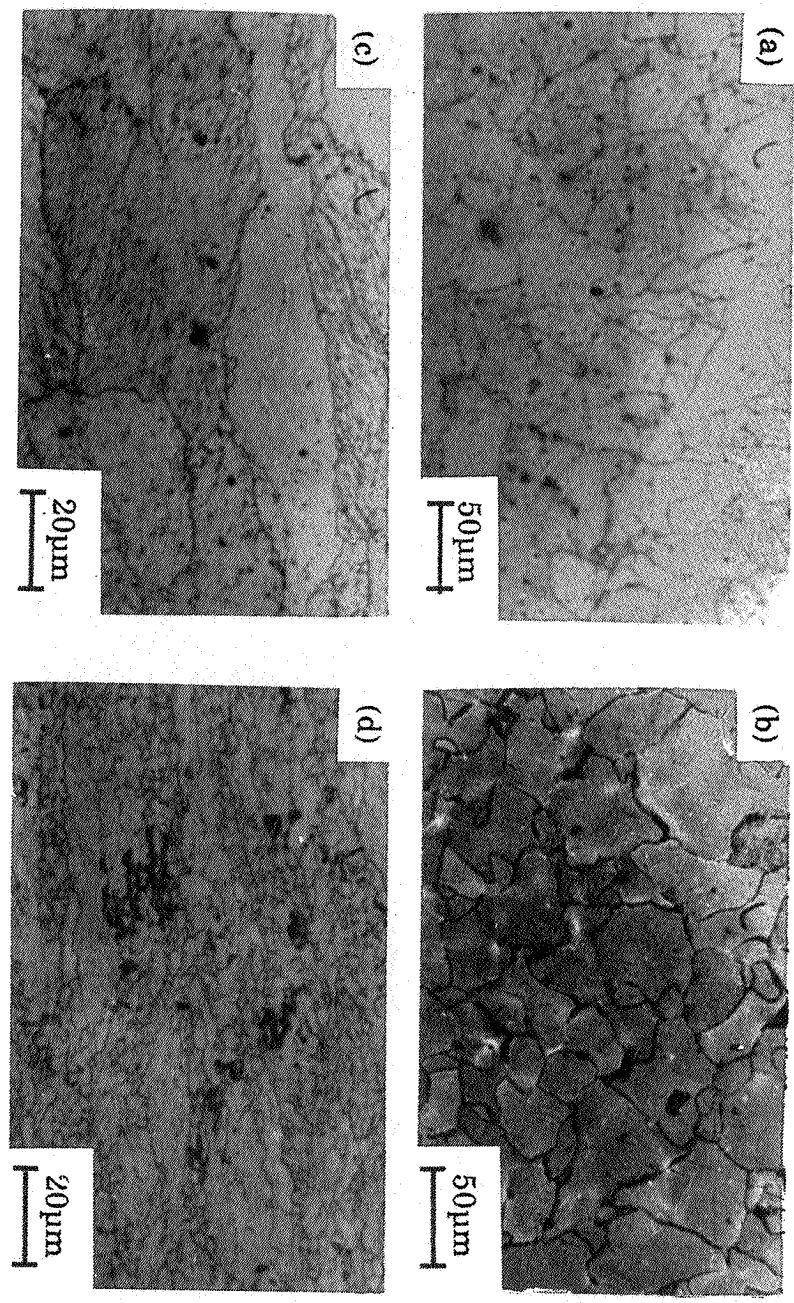
شکل ۱۰ - تغییرات ریزساختار فولاد (C ۰/۰۷۵) منگامی که در دمای ۶۵۰°C و در سرعت کرنش ۱/۲ قبل از تغییر فرم (b) در کرنش ۰/۲ (c) در کرنش ۰/۴ (d) در کرنش ۱/۲ \times 10^{-3}s^{-1} تغییر فرم یافته است.
