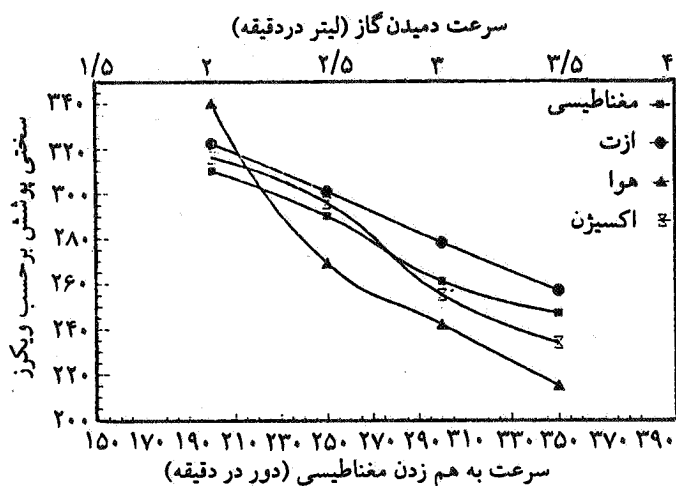
شکل ۵- تأثیر میزان به هم زدن حمام روی سختی پوشش کامپوزیتی Ni-P-MoS 2 در حمامی با بارگذاری ۱۰ گرم در لیتر
