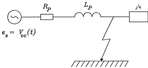
شکل ۲- وقوع اتصال کوتاه سه فاز متقارن در یک شبکه قدرت ساده
