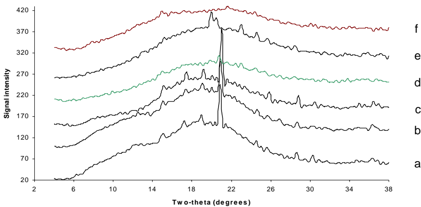
نمودار ۴. الگوی دیفرکسیون X-ray نمونه‌های انجیر تیمار یافته با ۰/۴۰ گلوکز سیراب به تعادل رسیده در فعالیت آبی‌های (a: ۰/۱۱۲، b: ۰/۲۲۷، c: ۰/۳۸۲، d: ۰/۶۴۳، e: ۰/۷۴۳، f: ۰/۸۴۳) در دمای ۲۵ °C
