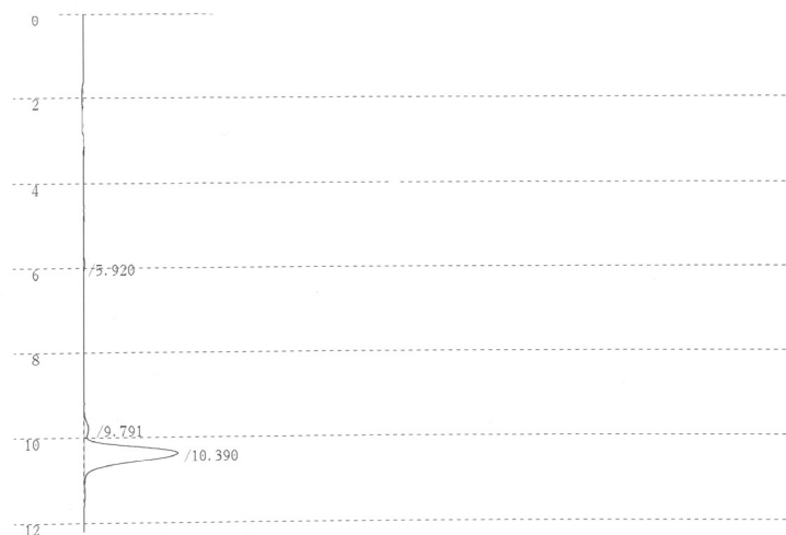
شکل ۱. کروماتوگرام مربوط به ترکیب استاندارد مونوآمونوم اسید گلیسریریزیکات (MAG) شرایط کروماتوگرافی: ستون RP-C_{18} (150 × 4.6 mm)، دمای آون 40^{\circ}C ، آشکار ساز UV (طول موج 254 nm)، فاز متحرک: متانول-آب-اسید استیک (۷۵V/V/V : ۲۴ : ۱)، سرعت جریان ۱ میلی لیتر در دقیقه
