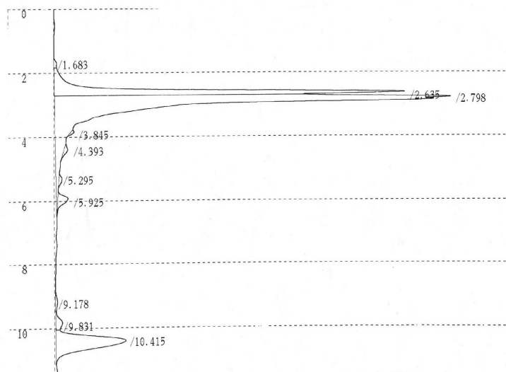
شکل ۲. کروماتوگرام HPLC عصاره ریشه شیرین بیان، شرایط کروماتوگرافی: ستون RP-C_{18} (150 × 4.6 mm)، دمای آون 40^{\circ}C ، آشکار ساز UV (طول موج 254 nm)، فاز متحرک: متانول-آب-اسید استیک (۷۵V/V/V : ۲۴ : ۱)، سرعت جریان ۱ میلی لیتر در دقیقه
