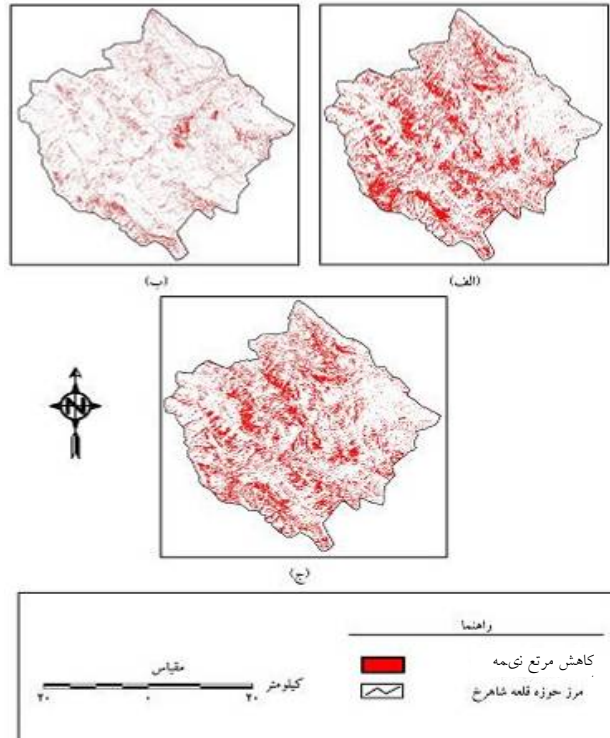
شکل ۷. روند کاهش مراتع نیمه انبوه طی سال‌های ۱۳۵۴ تا ۱۳۶۹ (الف)، ۱۳۶۹ تا ۱۳۸۱ (ب)، ۱۳۸۱ تا ۱۳۵۴ (ج).
