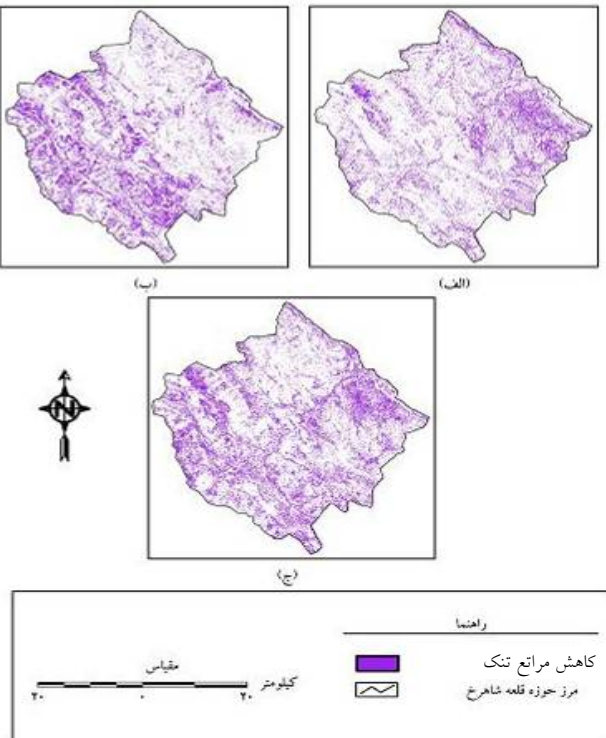
شکل ۸. روند کاهش مراتع تنک و اراضی با پوشش پراکنده طی سال‌های ۱۳۵۴ تا ۱۳۶۹ (الف)، ۱۳۶۹ تا ۱۳۸۱ (ب)، ۱۳۸۱ تا ۱۳۵۴ (ج).
