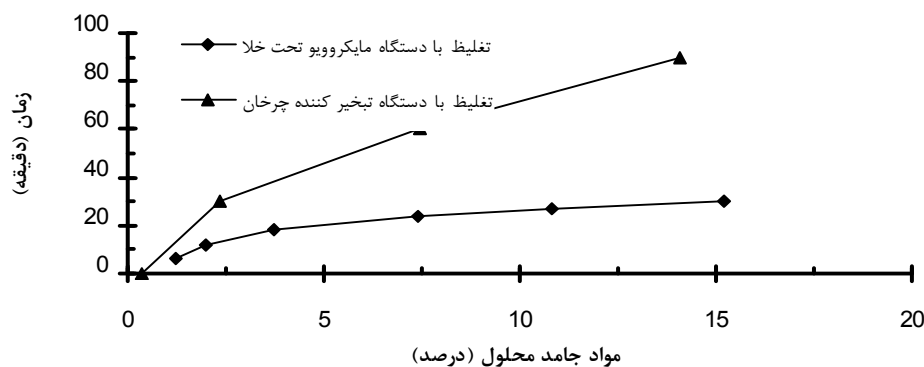
شکل ۲. مقایسه نمودارهای تغلیظ عصاره استخراجی کنگر فرنگی با استفاده از تبخیر کننده چرخان و مایکروویو تحت خلاء
