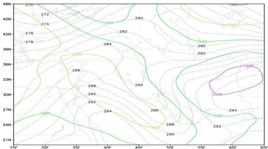
شکل ۱. نقشه همدیدی روز ۹ نوامبر ۱۹۹۶ ساعت ۱۲۰۰ UTC در تراز ۸۵۰ هکتوپاسکال
