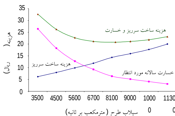
شکل ۴. برآورد هزینه‌های ساخت سرریز و خسارت مورد انتظار متناظر با گزینه‌های مختلف طراحی سرریز سد پیشین (روش مهندسين عمران)
