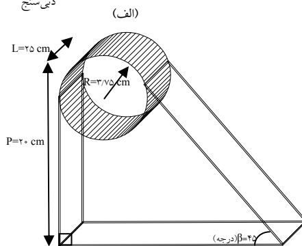
شکل ۳. الف) پلان مجموعه دستگاه آزمایش، ب) سرریز جانبی تاج دایره‌ای
