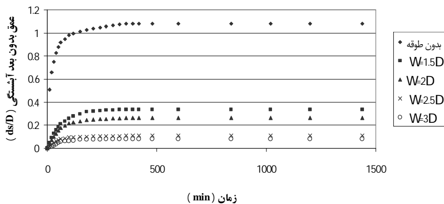
توسعه آبستگي برای طوق با ابعاد متفاوت در ارتفاع 0.5D زیر بستر
