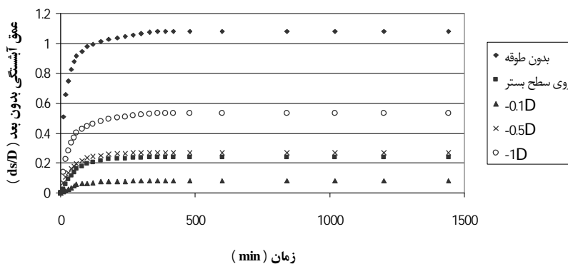
توسعه آبشستگی با طوق W=3D
