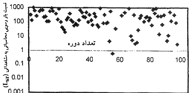
نمودار ۳-۱۰. روش فاضل، رودخانه کارون
