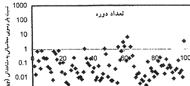
نمودار ۳-۴. روش توفالتی، رودخانه کارون
