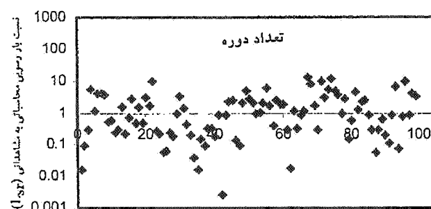
نمودار ۲-۴. روش توفالتی، رودخانه کرخه
