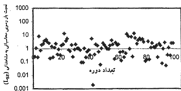
نمودار ۷-۲. روش انگلاند و هانسن، رودخانه کرخه
