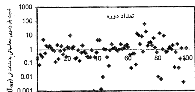
نمودار ۸-۲. روش یانگ، رودخانه کرخه
