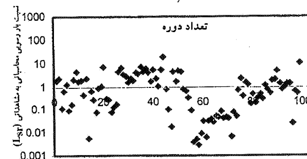
نمودار ۸-۳. روش یانگ، رودخانه کارون
