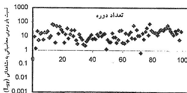
نمودار ۱-۶. روش وایف، رودخانه دز
