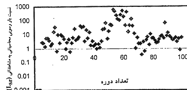
نمودار ۸-۱. روش یانگ، رودخانه دز
