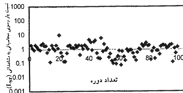
نمودار ۷-۳. روش انگلاند و هانسن، رودخانه کارون
