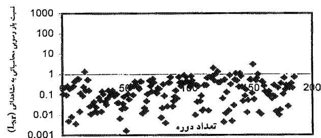
نمودار ۷-۲. روش انگلاند و هانسن، رودخانه کرخه
