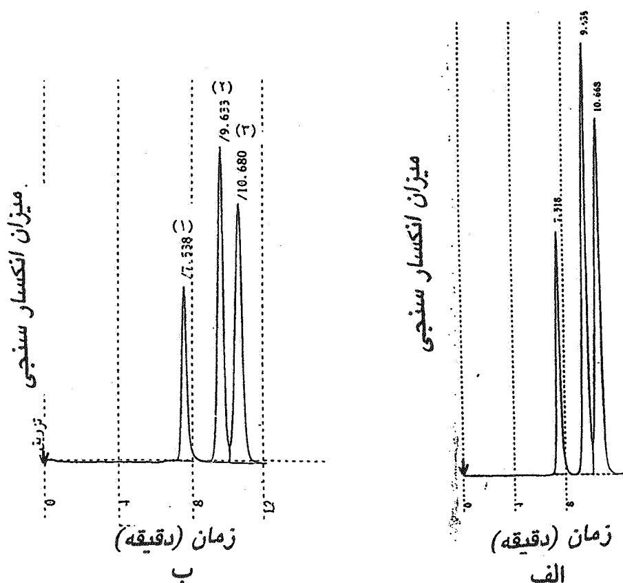
شکل ۱. کروماتوگرام قندهای گلوکز، فروکتوز و ساکارز (الف) نمونه استاندارد و ب) نمونه سیب زمینی آگریا در هفته پانزدهم، تجزیه شده با کروماتوگرافی مایع با کارایی زیاد، با زمان ماندگاری: ساکارز ۷/۵ دقیقه، گلوکز ۹/۶ دقیقه و فروکتوز ۱۰/۷ دقیقه
