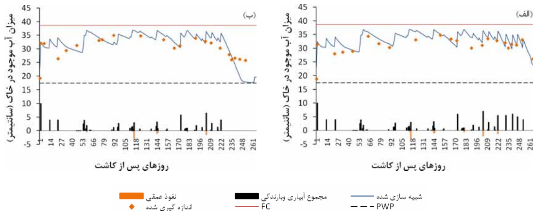
شکل ۳. مقادیر اندازه‌گیری شده آب خاک در مقابل مقادیر شبیه‌سازی شده الف: I ۱ - ب: I ۲ (سری داده‌های مستقل شعبانی و همکاران (۵))
