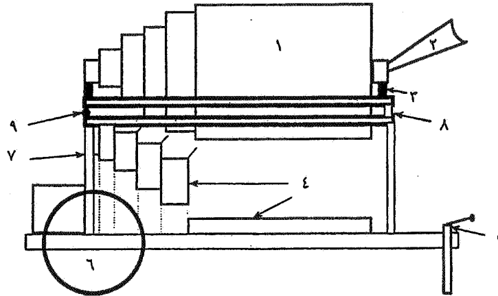
۱- مجموعه الکهای دوار ۲- کانال تغذیه ۳- چرخهای لاستیکی ۴- مخازن خاکدانه ها ۵- چک ۶- چرخ حامل ۷- شاسی دستگاه ۸- پیچ تنظیم شیب ۹- لولا
