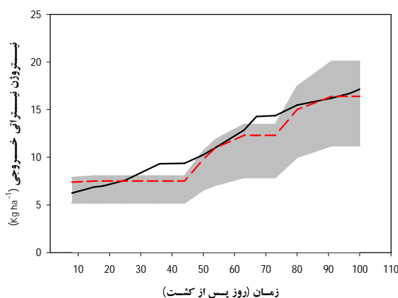
شکل ۴. نتایج شبیه‌سازی نیتروژن نترات آیشویی شده برای شرایط عدم کاربرد C_p (کنترل): داده‌های مشاهده‌ای (خط) و بهترین شبیه‌سازی (خط چین) و باند ۹۵PPU زه‌آب شبیه‌سازی شده (قسمت خاکستری).
