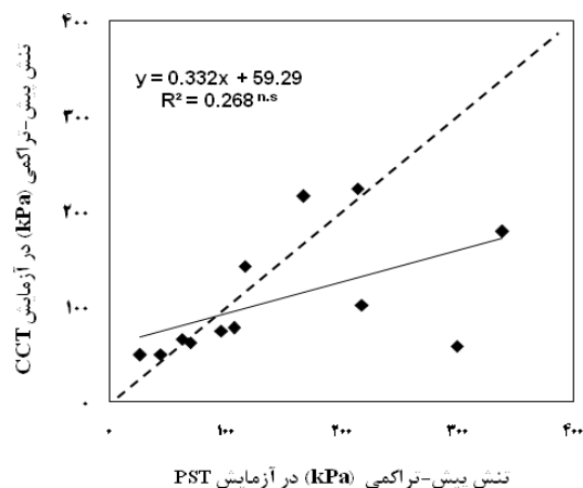
شکل ۶. رابطه‌ی بین میانگین مقادیر تنش پیش-تراکمی به‌دست آمده از روش کاساگراند در آزمایش‌های CCT و PST.
