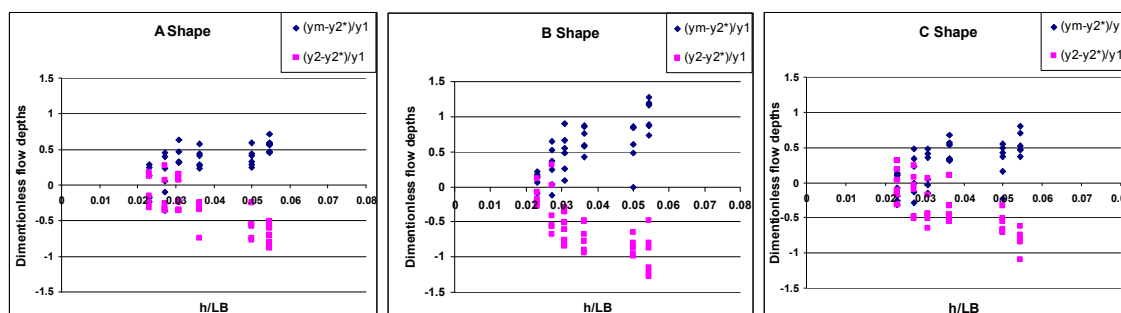
شکل ۳. تغییرات عمق آب قبل و بعد از آبپایه، به ترتیب از چپ به راست آبپایه کم عرض (مستطیلی) و آبپایه عریض (مربعی و پلکانی)
