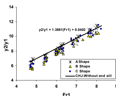
شکل ۱۰. مقایسه نسبت اعماق مزدوج پرش هیدرولیکی با بکارگیری آبپایه انتهایی
