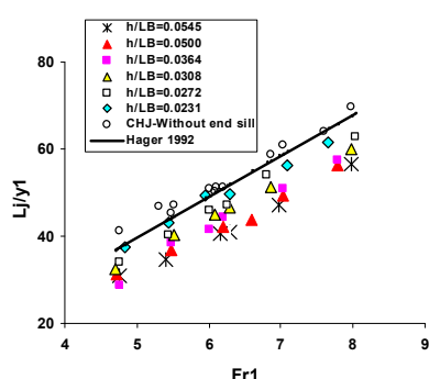
شکل ۱۲. مقایسه طول پرش هیدرولیکی، به ترتیب از چپ به راست آبپایه کم عرض (مستطیلی) و آبپایه عریض (مربعی و پلکانی)
