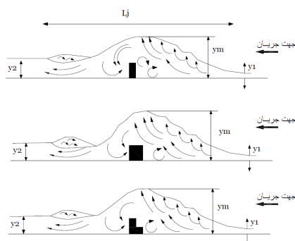
شکل ۱۴. نمایشی از تغییرات حجم پرش با سه شکل مختلف آبپایه
