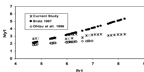
شکل ۷. مقایسه مقادیر آزمایشگاهی ارتفاع آبپایه برای قرار نگرفتن در حالت سرریزی
