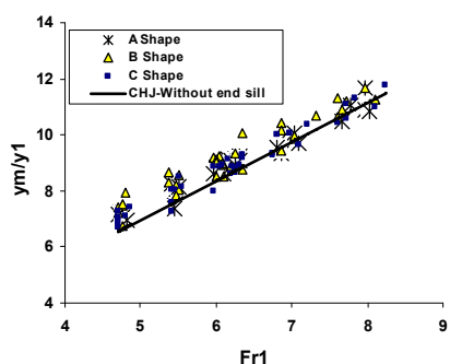
شکل ۱۱. مقایسه عمق نسبی ماکزیمم پرش هیدرولیکی با بکارگیری آبپایه انتهایی
