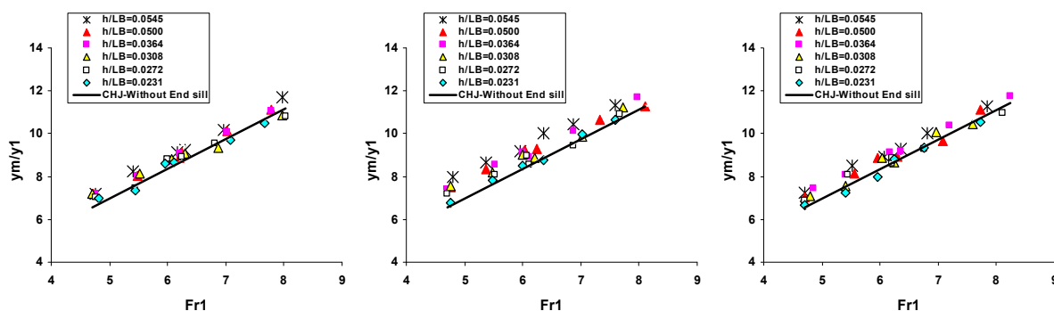
شکل ۸. مقایسه عمق نسبی ماکزیمم پرش هیدرولیکی،
