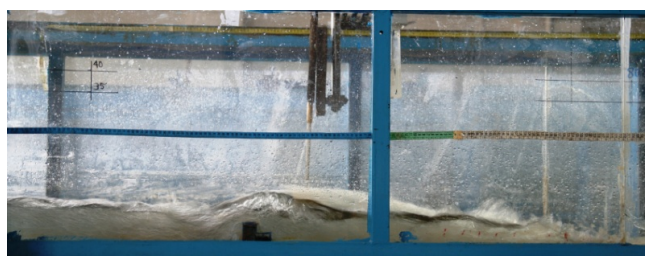
شکل ۶. پرش تثبیت شده توسط آبپایه انتهایی با مقطع عریض پلکانی ( L_B = 110\text{ cm} و h = 6\text{ cm} ، Fr_1 = 4/69 ، Q = 35\text{ LPS} )
