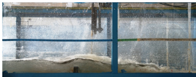
شکل ۴. پرش تثبیت شده توسط آبپایه انتهایی با مقطع کم عرض مستطیلی ( L_B = 110\text{ cm} و h = 6\text{ cm} ، Fr_1 = 4/76 ، Q = 35\text{ LPS} )
