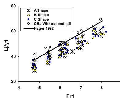
شکل ۱۳. مقایسه طول پرش هیدرولیکی با بکارگیری آبپایه انتهایی
